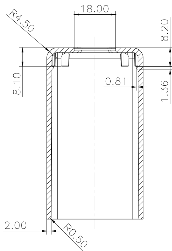
Section D-D
